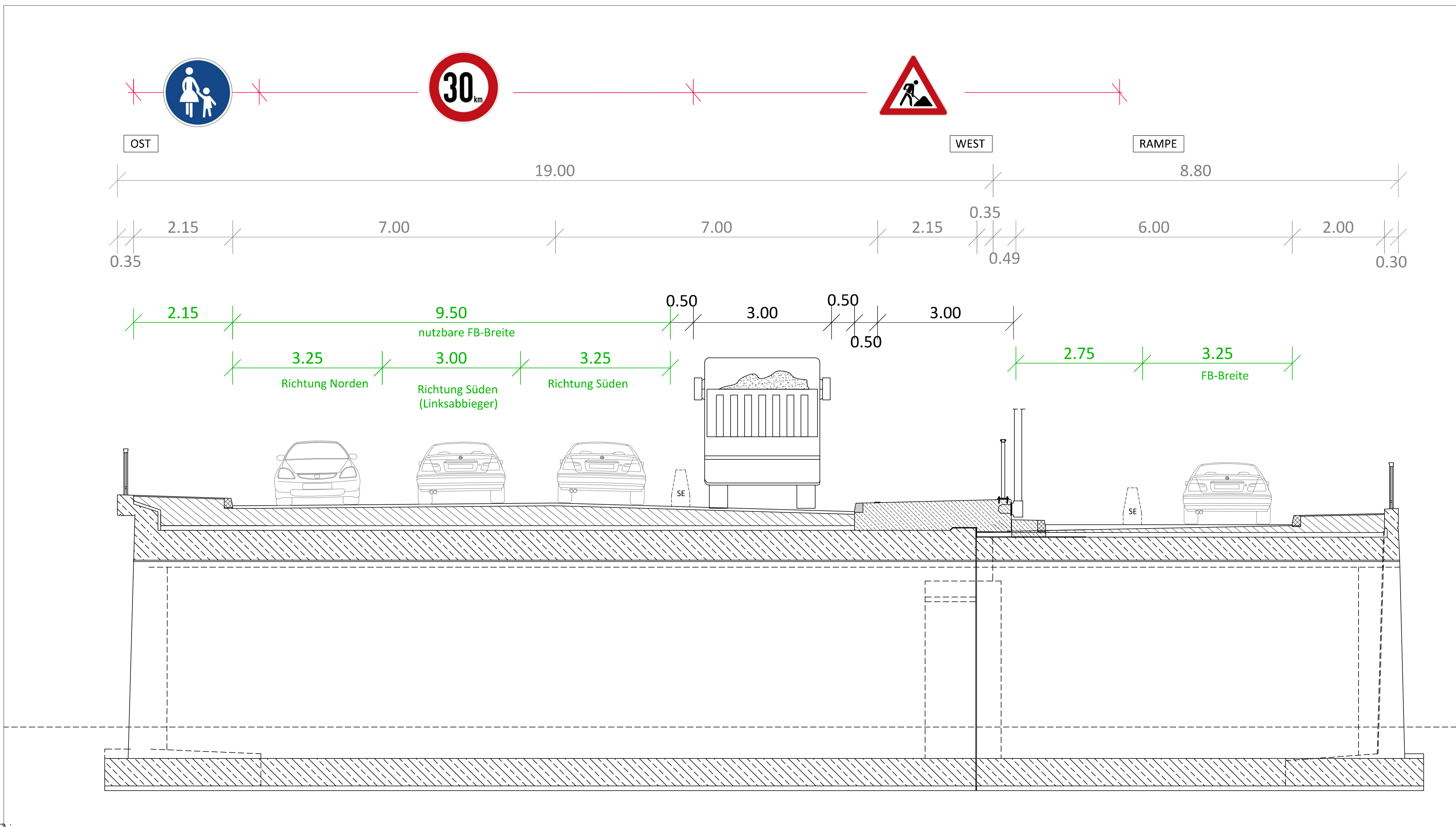
Schnitt 1-1 - M 1: 50 Bauzeitliche Verkehrsführung Kappenerneuerung Stützwände, Angerbadergasse Westseite - Bauphase 1a
