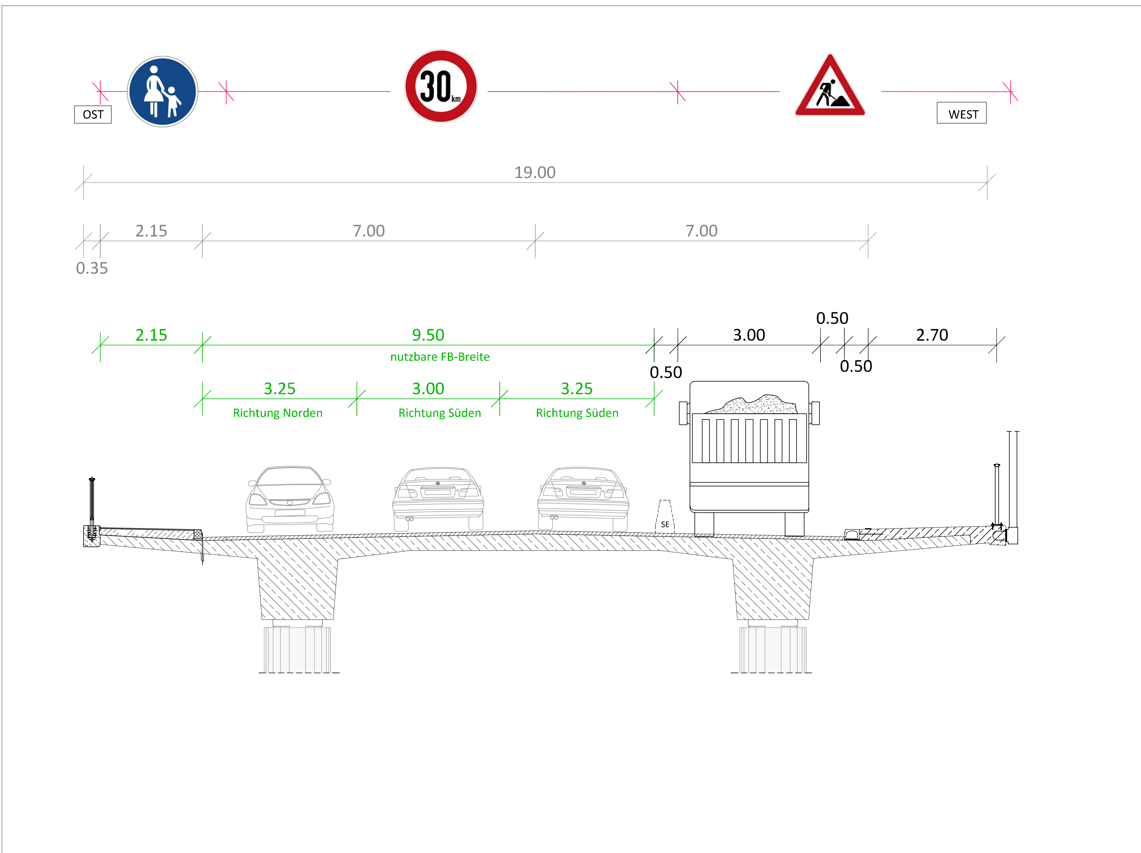
Schnitt 2-2 - M 1:50 Bauzeitliche Verkehrsführung Kappenerneuerung Hochtrasse Westseite - Bauphase 1a
